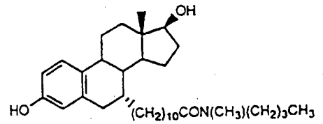
ICI 164384
